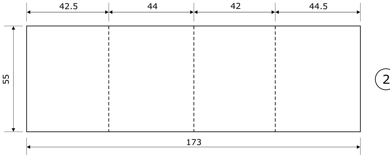
Plano # 1 de despiece y plantillas de construcción de bastidor para transformador. REF: 38 mm x 40 mm 231 watts
