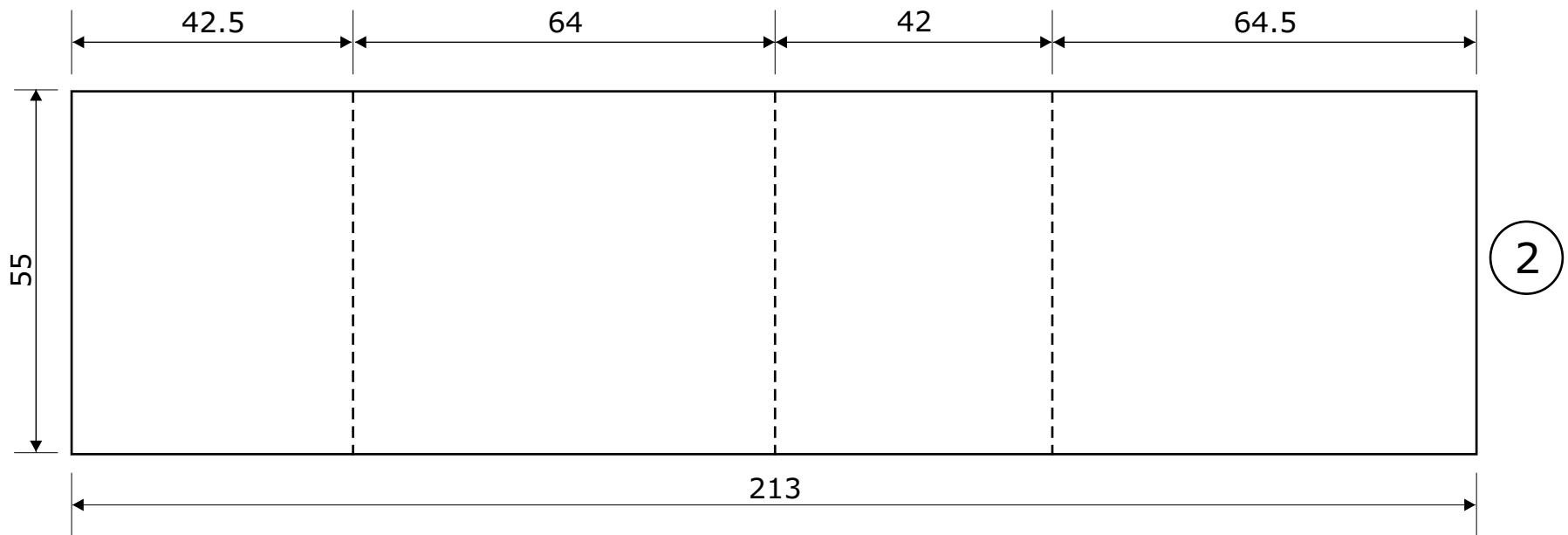
Plano # 1 de despiece y plantillas de construcción de bastidor para transformador. REF: 38 mm x 60 mm 231 watts
