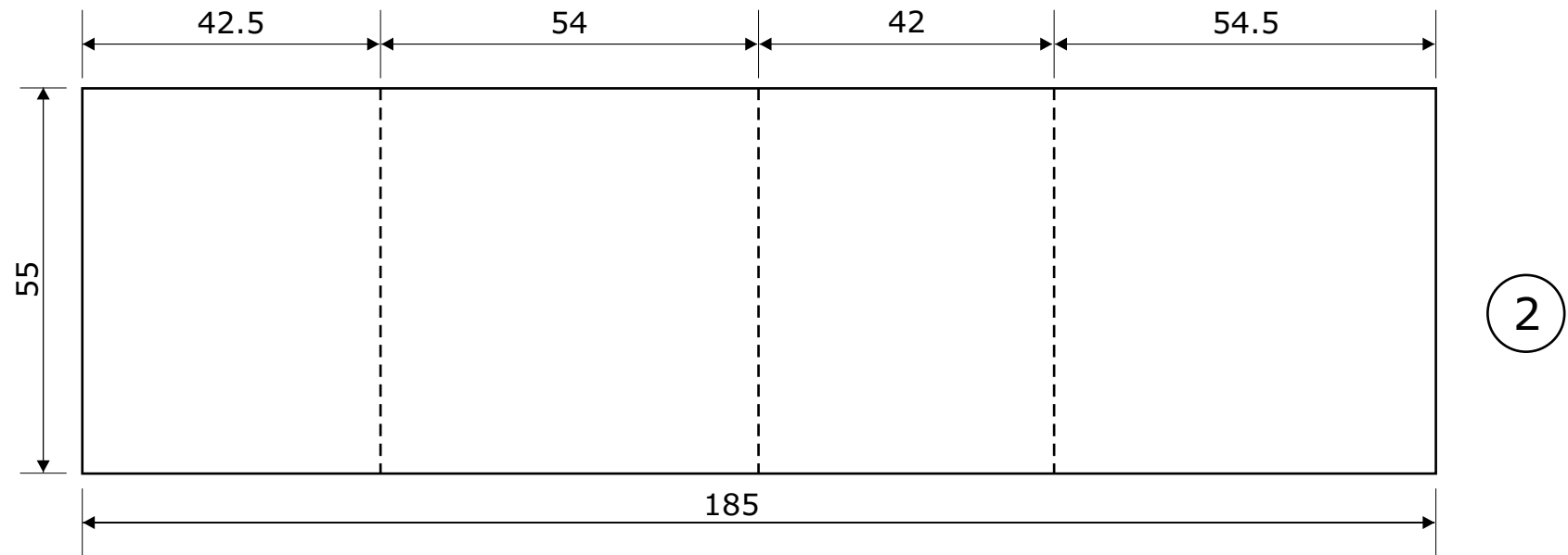
Plano # 1 de despiece y plantillas de construcción de bastidor para transformador. REF: 38 mm x 50 mm 231 watts
